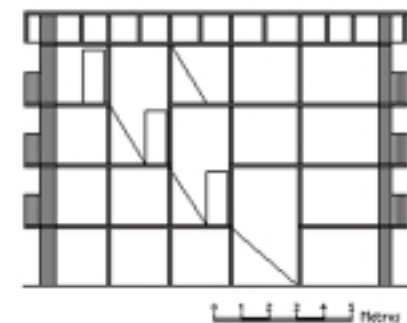
Bermeoko arrantzaleen etxea. Profila eta aurrealdea (A.A).
